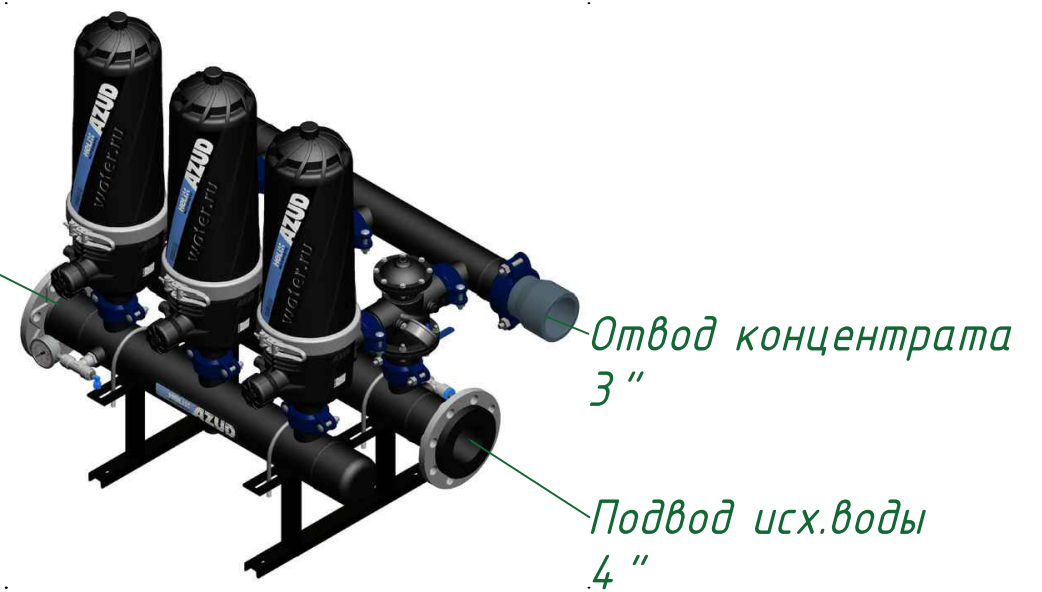
Изометрия
